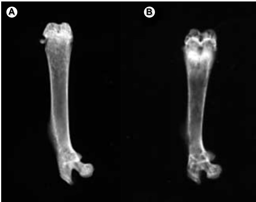
Figure 3. Radiographies du fémur d'animaux déficients pour le gène de la 25-hydroxyvitamine D-1 \alpha -hydroxylase (1 \alpha -OHase). A. Fémur d'un animal hétérozygote. B. Fémur d'un homozygote mutant pour la 1 \alpha -OHase. Notez l'élargissement de la plaque de croissance et la minceur du cortex du fémur mutant, démontrant la présence de rachitisme et d'ostéomalacie.
