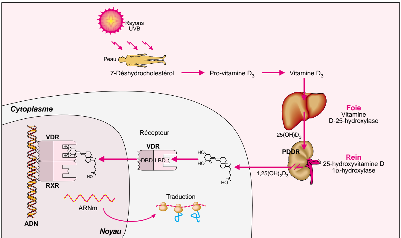
Figure 1. Biosynthèse de la 1,25(OH) 2 D 3 . La vitamine D (ici D 3 puisque le schéma s'applique à l'homme), synthétisée suite à l'irradiation de la peau par les rayons solaires, est convertie en 25-hydroxyvitamine D 3 [25(OH)D 3 ] par la vitamine D 25-hydroxylase au niveau du foie. Ce métabolite inactif est ensuite métabolisé en 1 \alpha ,25-dihydroxyvitamine D 3 [1,25(OH) 2 D 3 ] à la suite de l'action de l'enzyme rénale, la 25-hydroxyvitamine D-1 \alpha -hydroxylase (1 \alpha -OHase). L'hormone 1,25(OH) 2 D 3 se lie ensuite à son récepteur nucléaire, le VDR (vitamin D receptor), un récepteur nucléaire de type II qui forme un dimère actif avec son partenaire, le RXR (retinoid X receptor), et module la transcription de gènes cibles. Le ligand du RXR, l'acide 9-cis rétinolique, n'est pas illustré. La cause moléculaire des rachitismes PDDR (pseudo vitamin D deficiency rickets), – des mutations dans le gène codant pour la 1 \alpha -OHase – est illustrée par la flèche interrompue au niveau du rein. L'autre forme de rachitisme héréditaire vitamino-dépendant, HVD-RR (hereditary vitamin D resistant rickets), est due à des mutations affectant la structure ou la fonction du VDR, soit au niveau du domaine de liaison du ligand (LBD, ligand binding domain), soit au niveau du domaine de liaison à l'ADN (DBD, DNA binding domain).
