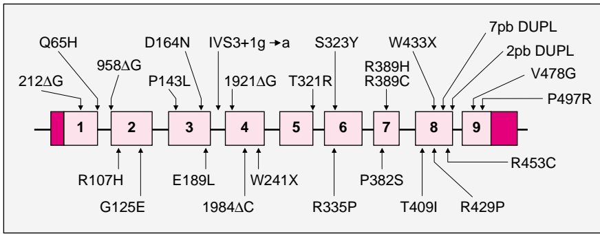
Figure 2. Mutations chez les patients atteints de rachitisme PDDR (pseudo-vitamine D deficiency rickets). La structure du gène de la 25-hydroxyvitamine D-1 \alpha -hydroxylase (1 \alpha -OHase) est représentée de façon schématique. Les exons sont numérotés de 1 à 9; les régions rouges correspondent aux séquences non-traduites en 5' et en 3', respectivement. Les 26 mutations identifiées jusqu'à présent chez des patients atteints de rachitisme PDDR sont représentées au-dessus et en dessous de la carte du gène. Les nombres indiquent le nucléotide ou l'acide aminé muté, selon le cas. \Delta : délétion; IVS3 + 1g \rightarrow a: mutation dans l'intron 3 (intervening sequence 3) affectant l'épissage; 7 bp dupl: duplication de 7 paires de bases; 2 pb dupl: duplication de 2 paires de bases.
