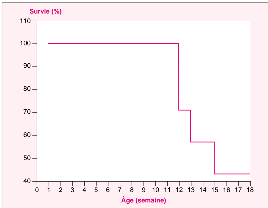
Figure 4. Survie des homozygotes mutants pour le gène de la 25-hydroxyvitamine D-1 \alpha -hydroxylase (1 \alpha -OHase). Les souris déficientes pour le gène 1 \alpha -OHase ont été sevrées à l'âge de trois semaines et alimentées par un régime normal. Dans ces conditions, les animaux meurent entre la 11 e et la 16 e semaine de vie.
