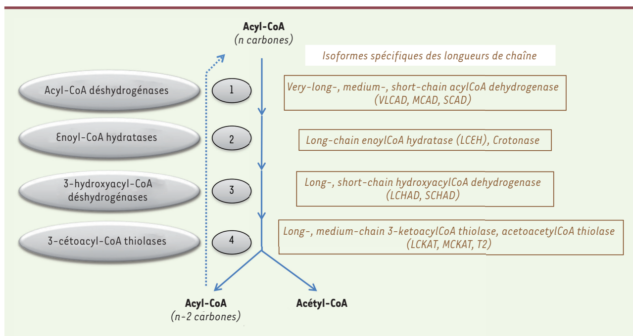
Figure 2. Étapes enzymatiques de l'hélice de Lyon.
