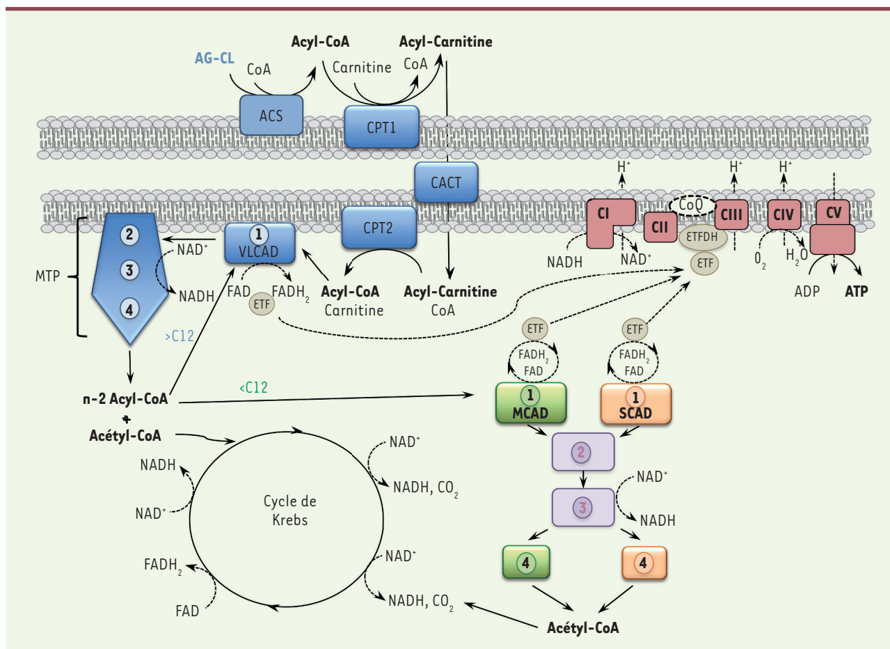
Figure 1. Organisation schématique de la \beta -oxydation mitochondriale des acides gras. Les acides gras à chaîne longue (AG-CL) activés en acyl-CoA par l'ACS (acyl-CoA synthetase) sont pris en charge par la navette d'import mitochondriale constituée de la CPT1 (carnitine palmitoyl transferase 1), de la CACT (carnitine acyl-carnitine translocase) et de la CPT2 (carnitine palmitoyl transferase 2), dont le fonctionnement dépend de la carnitine. Les chiffres 1 à 4 correspondent aux quatre étapes de l'hélice de Lén. À l'intérieur de la mitochondrie, les acyl-CoA sont oxydés par la VLCAD (very-long-chain acyl-CoA dehydrogenase) (étape 1) puis par la MTP (mitochondrial trifunctional protein) (étapes 2, 3, 4) aboutissant à la formation d'un acyl-CoA raccourci de deux carbones ( n-2 acyl-CoA), d'un acétyl-CoA, d'un NADH, et d'un FADH 2 . Cette séquence se reproduit à l'identique jusqu'à l'obtention d'un acyl-CoA à chaîne moyenne (12 carbones) qui sera dirigé vers la MCAD (medium chain acyl-CoA dehydrogenase) (étape 1) puis vers des isoformes communes aux chaînes moyennes et courtes pour les étapes 2 et 3, et, enfin, vers l'isoforme spécifique des chaînes moyennes en étape 4. Une fois réduit à 6 carbones, l'acyl-CoA réagira finalement avec la SCAD (short chain acyl-CoA dehydrogenase) (étape 1) puis avec les isoformes communes des étapes 2 et 3, et avec l'isoforme spécifique des chaînes courtes à l'étape 4. La conversion complète d'un AG-CL en acétyl-CoA mobilise donc successivement toutes les isoformes enzymatiques (chaîne longue, moyenne et courte). Le fonctionnement de la \beta -oxydation est étroitement couplé à l'activité de la chaîne respiratoire, permettant la production de grandes quantités d'ATP. Les électrons du FADH 2 produits à l'étape 1, d'abord cédés à l'ETF (electron-transferring factor) sont introduits dans la chaîne respiratoire via un accepteur spécifique, l'ETF-DH (electron-transferring factor dehydrogenase). Le NADH produit au cours de la \beta -oxydation des acides gras alimente la chaîne respiratoire au niveau du complexe I.
