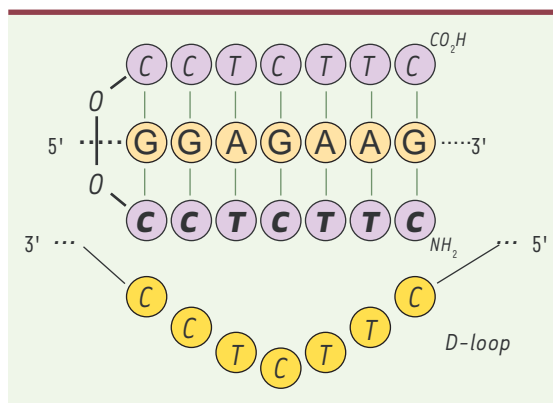
Figure 3. Structure en triple hélice (PNA) 2 /DNA. L'hybridation de deux molécules de PNA avec un brin d'ADN complémentaire entraîne le déplacement de l'autre brin d'ADN qui va ainsi former une boucle d'ADN simple brin (D-loop). Dans le triplex formé entre les deux PNA et le brin d'ADN, l'un des brins PNA est lié à l'ADN par des liaisons hydrogènes classiques de type Crick et Watson, et l'autre par des liaisons hydrogènes de type Hoogsteen (les liaisons entre les bases sont représentées par des traits verts).
